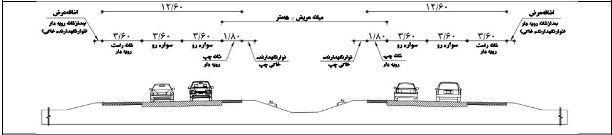
F۱۰- آزادراه چهار خطه با DDHV برابر و بیشتر از ۲۵۰ با میانه عریض
