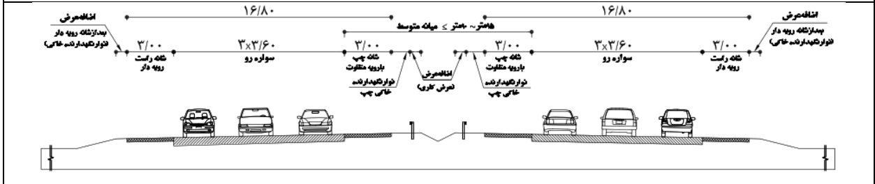
F۱۱- آزادراه شش خطه با DDHV کمتر از ۲۵۰ با میانه متوسط
