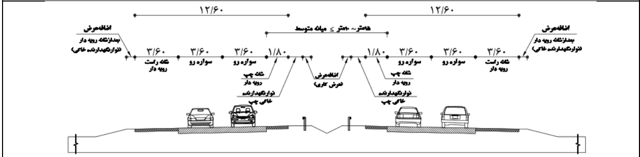
F۹- آزادراه چهار خطه با DDHV برابر و بیشتر از ۲۵۰ با میانه متوسط
