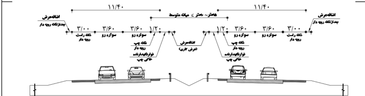
F۷- آزادراه چهار خطه با DDHV کمتر از ۲۵۰ با میانه متوسط
