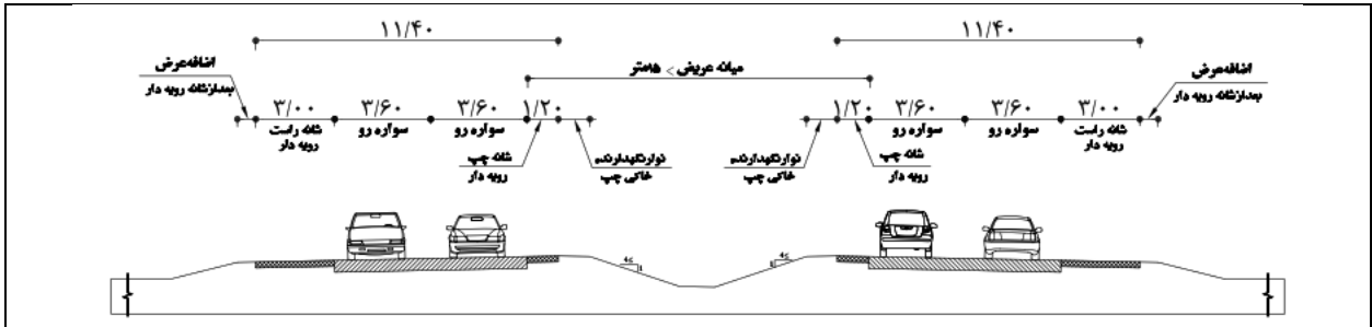
F۸- آزادراه چهار خطه با DDHV کمتر از ۲۵۰ با میانه عریض
